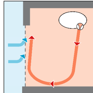
ADW-Einbau (Luftwalze nach außen drehend) ADW installation (outwards rotating air roll)
