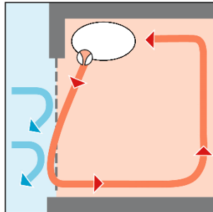
IDW-Einbau (Luftwalze nach innen drehend) IDW installation (inwards rotating air roll)
